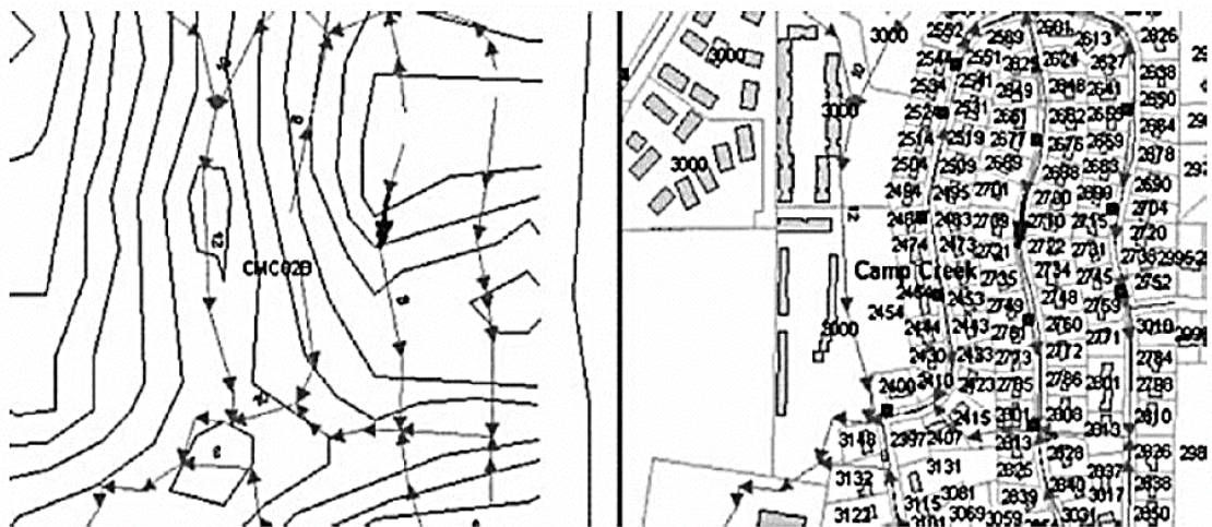
شکل ۲-۴ نمایش قسمت های طرح بهداشتی فاضلاب (الف) خطوط زمین (ب) خدمات پیوسته (Brown and Toomer ۲۰۰۳).
