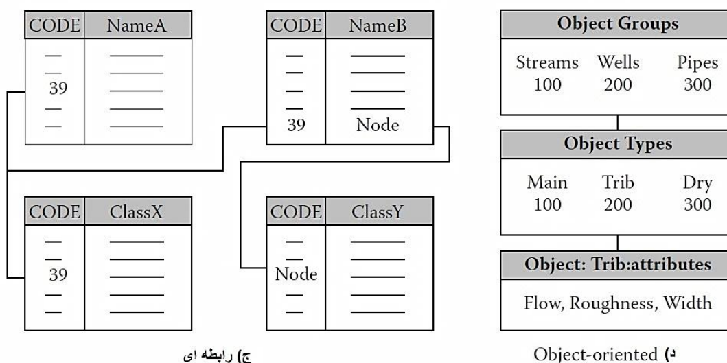
شکل ۳-۱۶ ساختار پایگاه داده.
