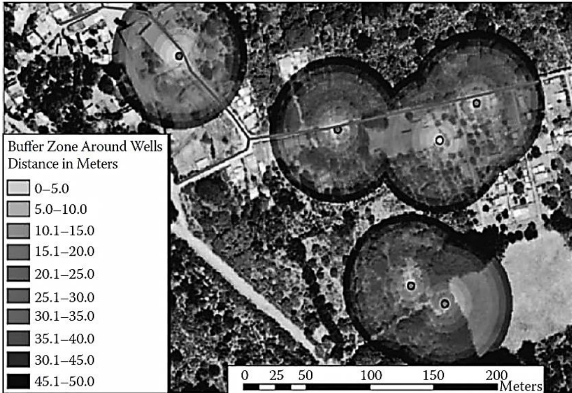
شکل ۴-۴ مثالی در موضوع عملیات بافر برای تعریف مناطق جهت حفاظت دهانه چاه از آلودگی.
