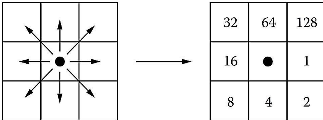
شکل ۴-۵ طرح جهت ۸D برای پردازش زمین.
