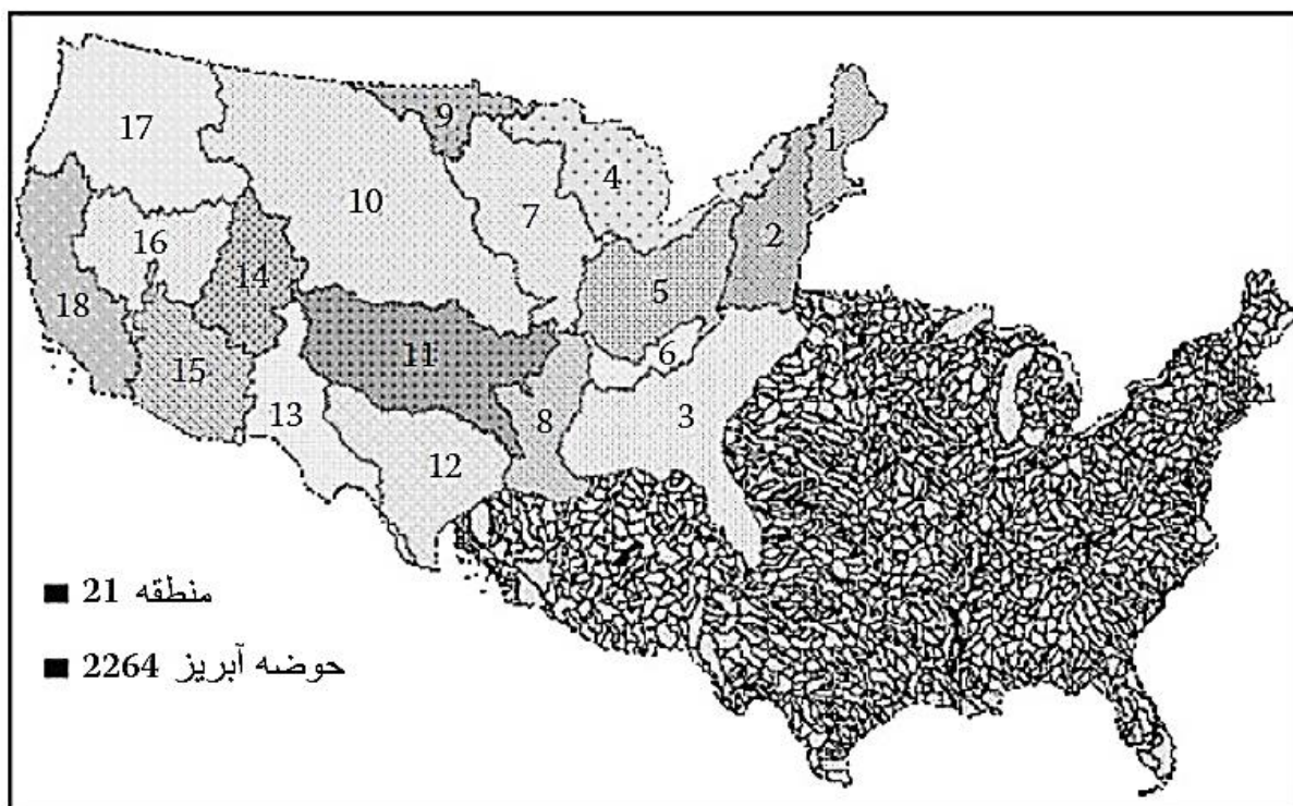
شکل ۳-۹ حوزه NHD در یک روش سلسله مراتبی برای سطوح مختلفی از مقیاس، سازمان یافته است (منبع: NHD ۲۰۰۰).
