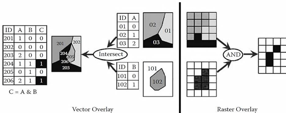
شکل ۱۰-۴ مثالی از عملیات همپوشانی رستری و برداری دو لایه از داده های ورودی.
