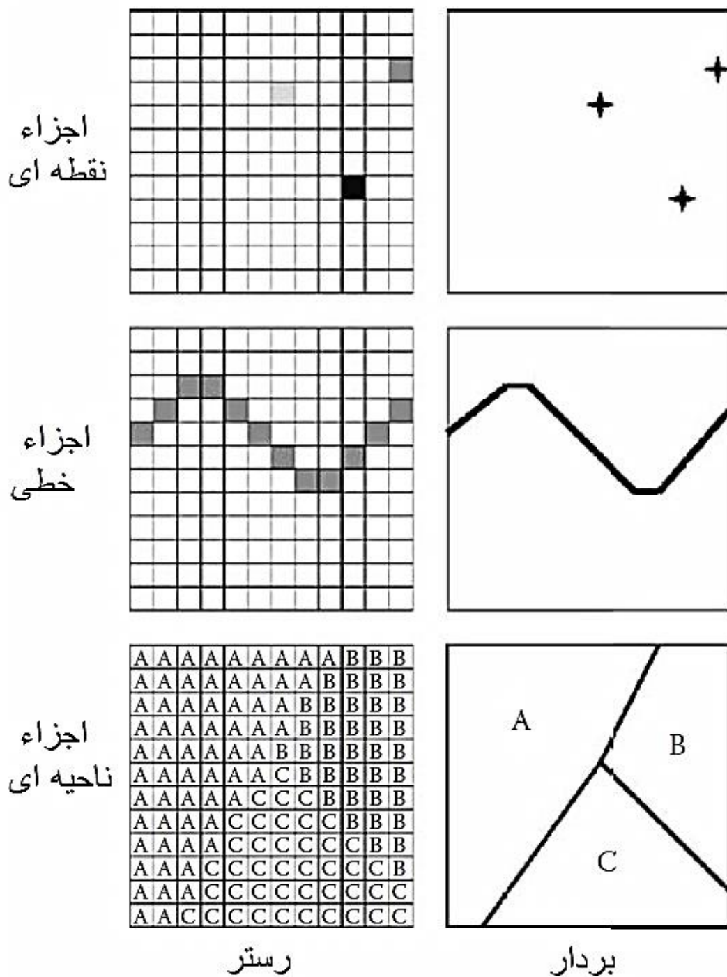
شکل ۵-۳ مدل داده های رستری و برداری؛ مدل داده های رستری توسط نقطه، خط و ناحیه هایی به عنوان مجموعه ای از سلول های با مقادیر معین نشان داده شده است.
